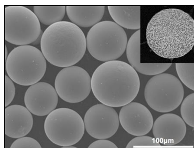
■ガスアトマイズ粉末の電子顕微鏡写真およびマイクロ組織
