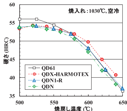
図2 焼入焼戻し硬さ
