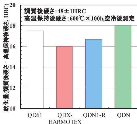
図4 軟化抵抗性
