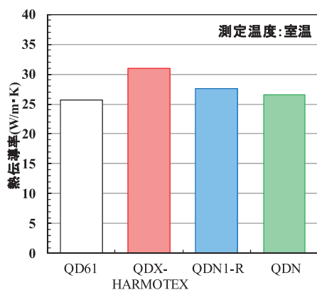
図5 熱伝導率
