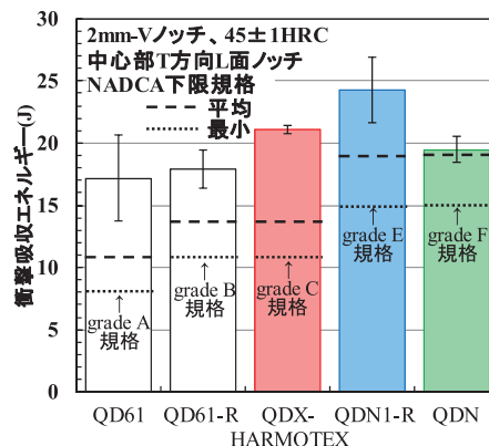
図3 シャルピー衝撃特性
