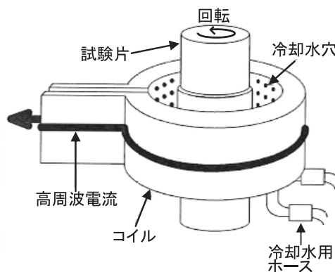
図6 ヒートチェック試験機概略図
