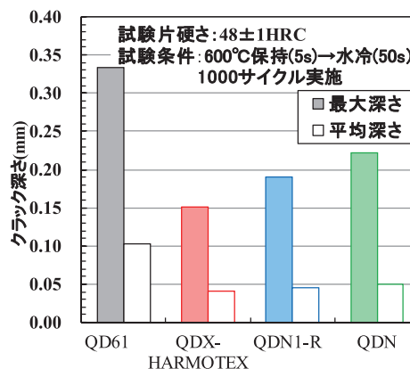
図7 ヒートチェック試験結果
